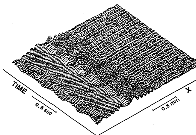
図5(b).Target Pattern 中心から発生する波動の伝搬の様子
