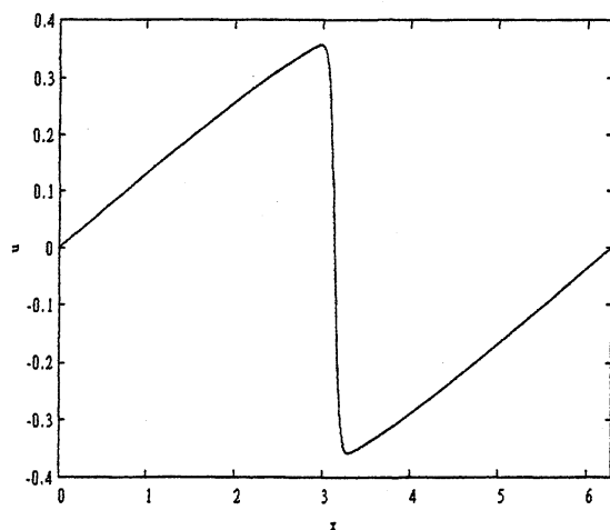
図1 バーガース方程式の速度分布( t=5 )
