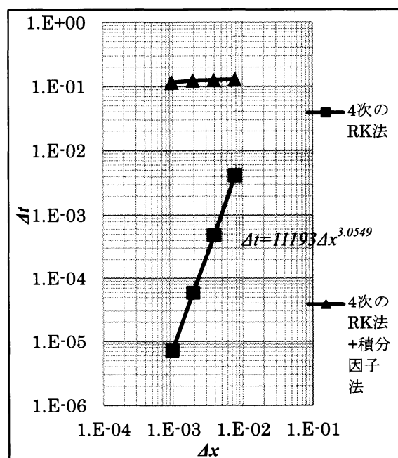
図6 \Delta x - \Delta t グラフ (KdV-バーガス方程式)
