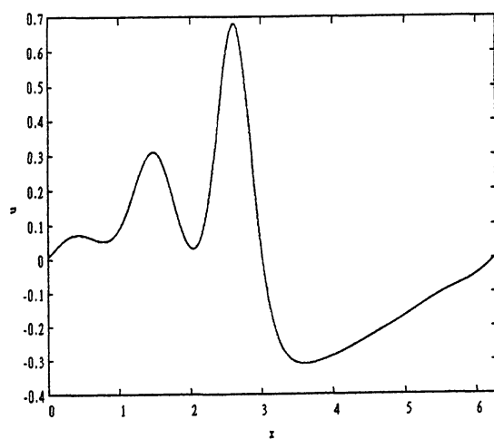
図5 KdV-バーガス方程式の速度分布( t=5 )
