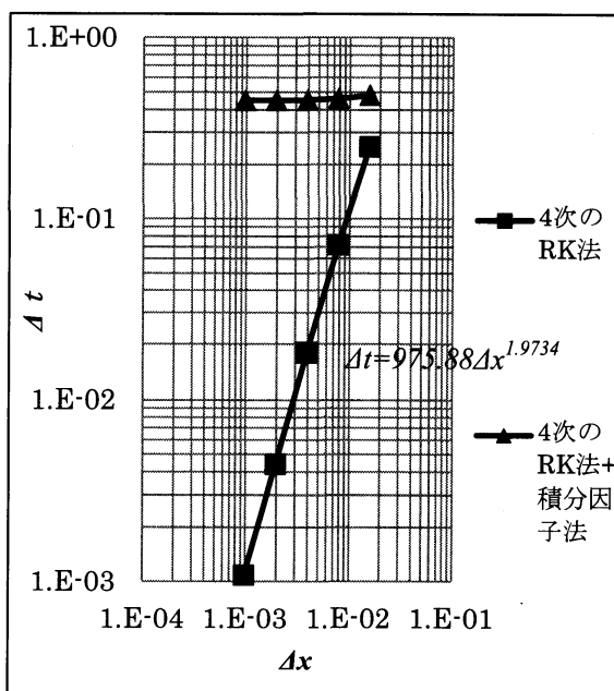
図2 \Delta x - \Delta t グラフ (バーガース方程式)
