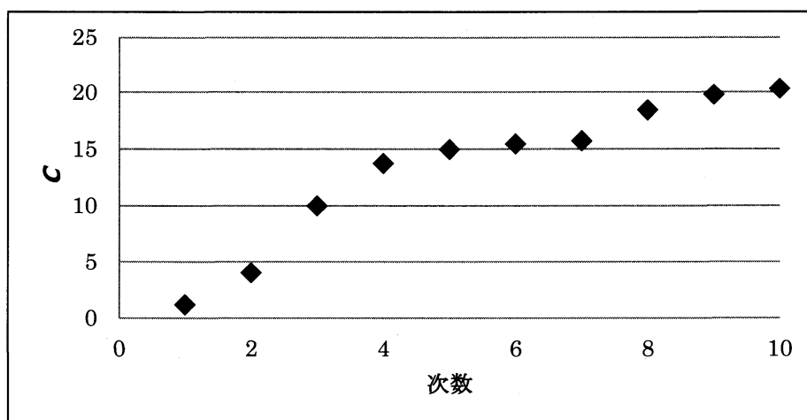
図9 次数と数値安定性
