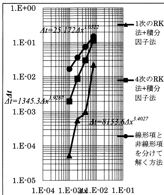
図8 \Delta x - \Delta t グラフ (5th KdV 方程式)
