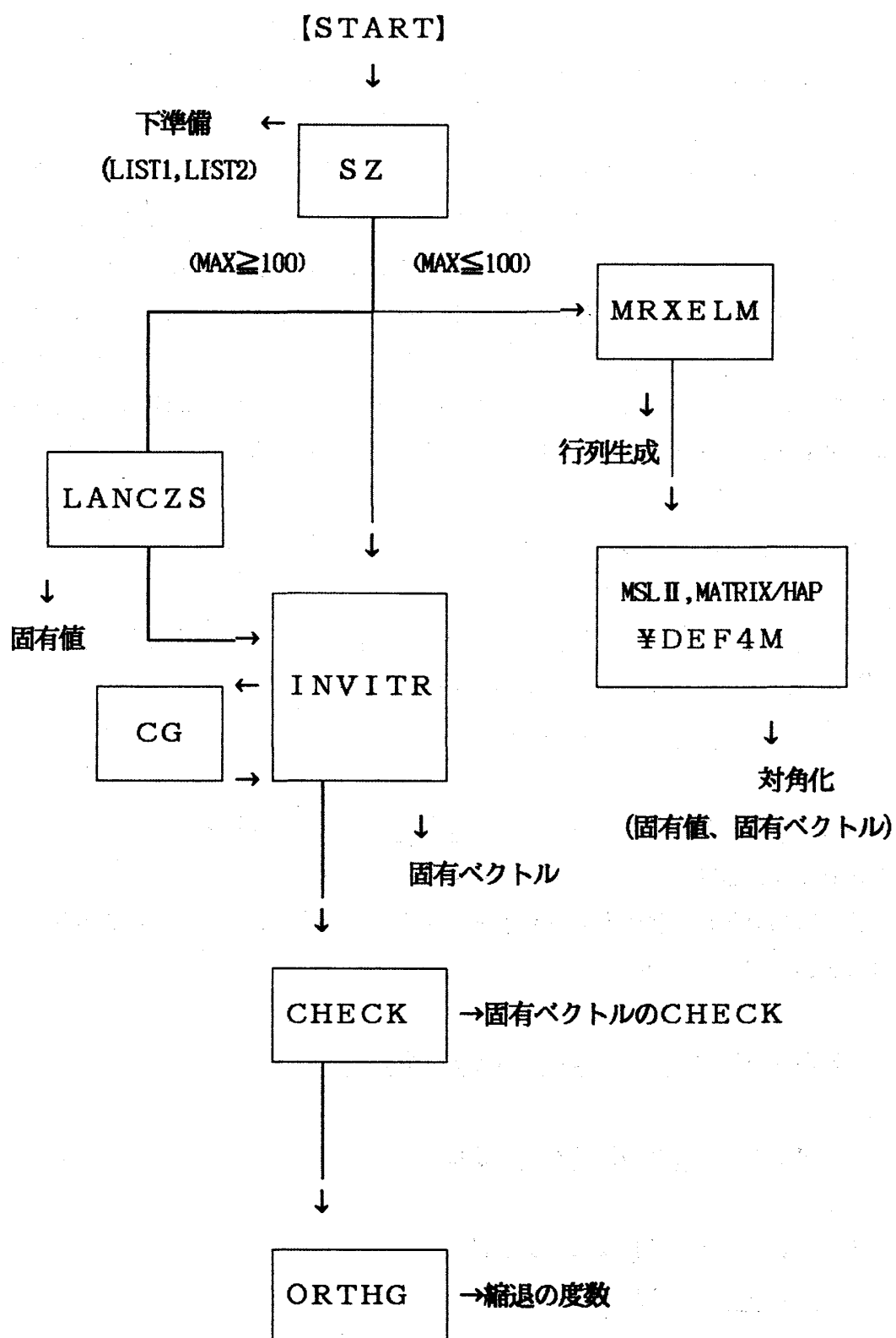
Fig. 1 TITPACK 流れ図
