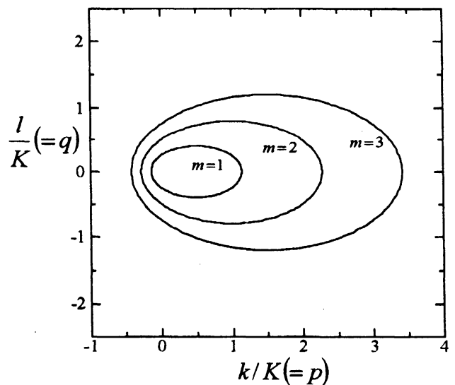
図 3 (1.8) で表される共鳴曲線 ( m=1,2,3 ). a=0.7 の例.
