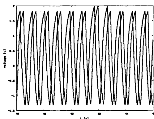
図 1: 共通のランダム 2 値ノイズを加えることによる発信回路の同期。実験開始時(左図)には振動子の位相がずれているが、しばらくたつと(右図)位相がそろってくる。図にはそれぞれ 2 回の実験で得られた電圧信号が重ねて表示してある。
