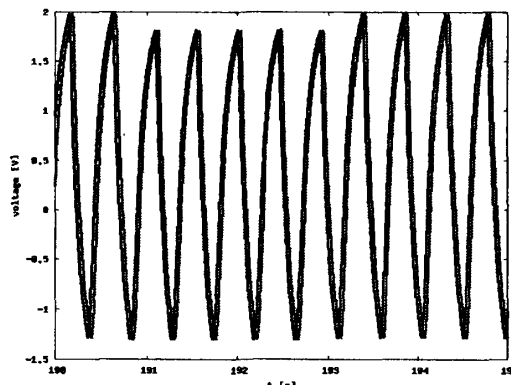
図 1: 共通のランダム 2 値ノイズを加えることによる発信回路の同期。実験開始時(左図)には振動子の位相がずれているが、しばらくたつと(右図)位相がそろってくる。図にはそれぞれ 2 回の実験で得られた電圧信号が重ねて表示してある。
