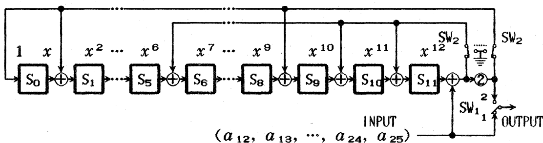
図 1 3 重誤り訂正 3 値 BCH (26, 14) 符号回路
