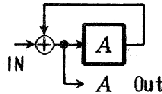
図 5 A 計算回路 Fig.5 An A generator.
