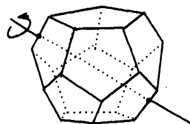
2 回の対称軸
