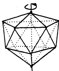
5 回の対称軸
