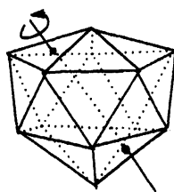
3 回の対称軸
