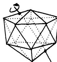
2 回の対称軸
