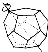
3 回の対称軸
