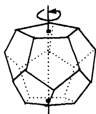
5 回の対称軸
