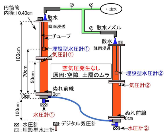
図 5.13 円筒管内状況 (幅下(2022 に加筆))
