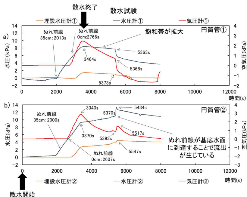
図 5.2 珪砂7号の実験結果(初期含水比 10%, 締固め回数1回)
