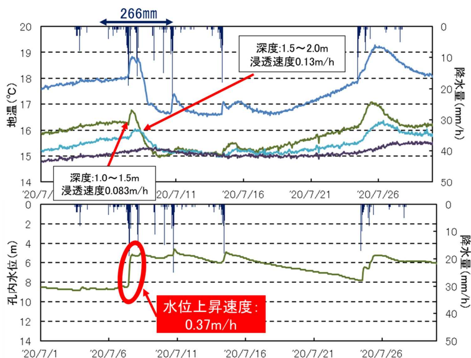
図 6.2 E7 における多層地温とボーリング孔 No.4 孔内水位の経時変化 (2020 年 7 月)
