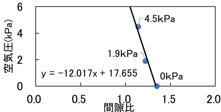
図 6.5 初期間隙比と間隙空気圧の上昇値の関係
