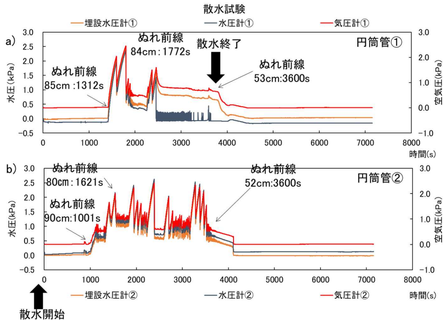
図 5.4 珪砂 8 号の実験結果(初期含水比 10%, 締固め回数 1 回)
