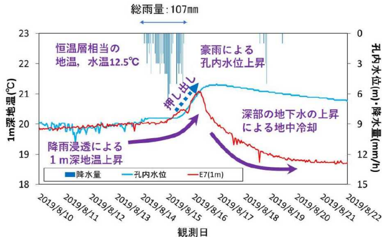
図 7.1 異常地温発生時における深部地下水の押し出し
