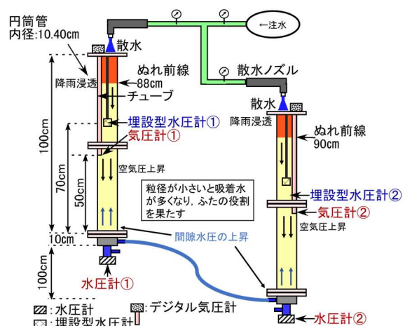
図 5.9 間隙空気圧と間隙水圧が上昇時に
