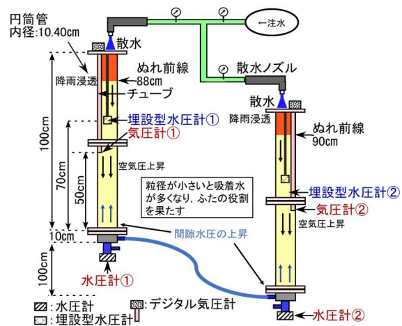
図 5.5 間隙空気圧と間隙水圧が上昇時における円筒管内状況
