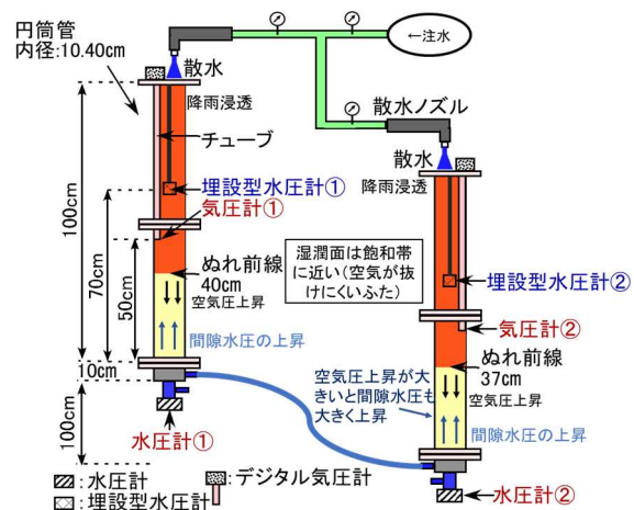
図 5.11 間隙空気圧と間隙水圧が上昇時に
