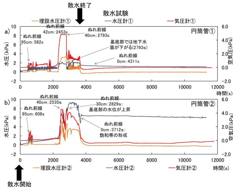
図 5.10 初期含水比 20%の実験結果(珪砂7号, 締固め回数1回)
