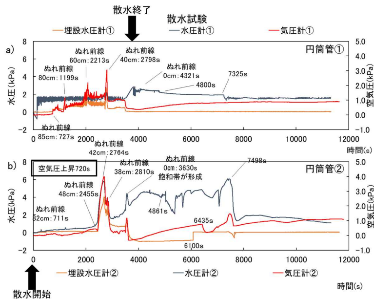
図 5.8 初期含水比 15%の実験結果(珪砂7号, 締固め回数1回)
