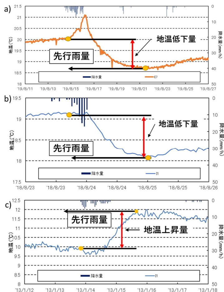
図 4.4 地温異常値とこれに伴う先行雨量の検討範囲の例(米田(2023 に加筆))
