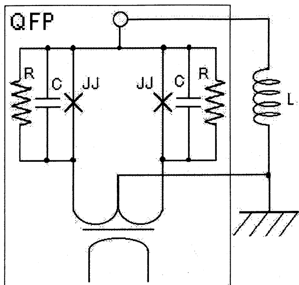
図 1. QFP 回路
