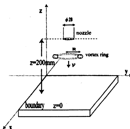
図 3: 座標系
