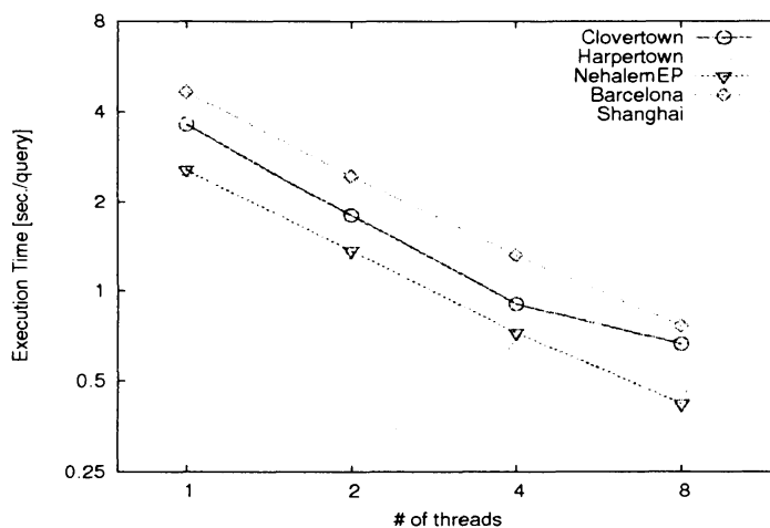
図 15: ダイクストラ法の実行時間 [秒/クエリ]
