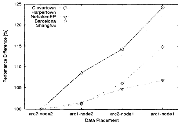
図 11: メモリ配置による性能差 [%]
