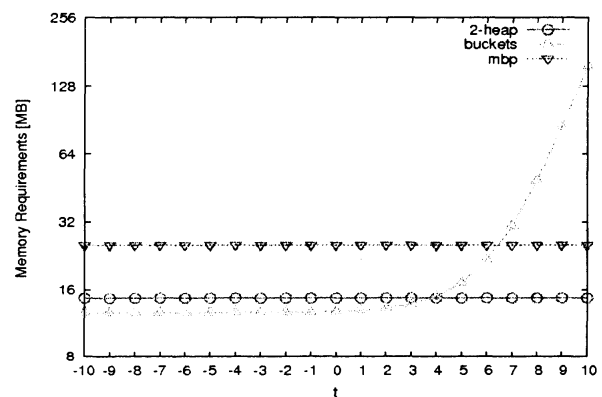
図2: 枝長スケーリングによるメモリ要求量の推移
