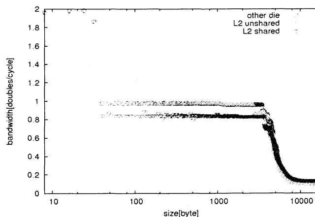
図 14: 2 プロセッサ・コア同時読み込みにおけるメモリ帯域幅 [doubles/cycle]
