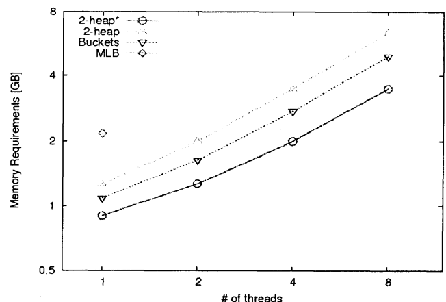
図 17: 優先キュー毎のメモリ要求量 [GB]
