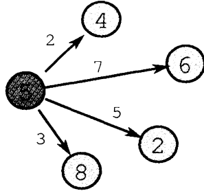
図 6: フォワードスター・グラフ表現
