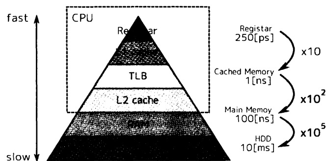
図 3: メモリ階層構造
