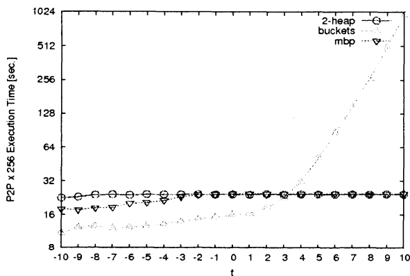
図1: 枝長スケーリングによる実行時間の推移
