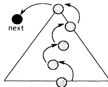
図 13: bottomup-extract-min
