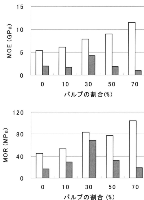
図8：樹皮粉末・パルプ成型物の強度特性 左：気乾、右：冷水浸漬
