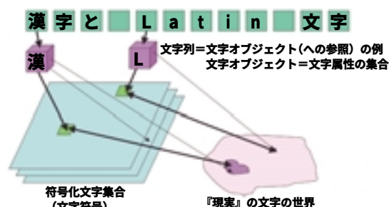
図2：UTF2000モデルの概念図
