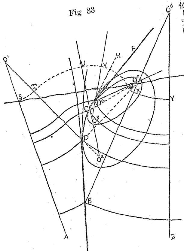
地質斷面圖の幾何學的作圖法
