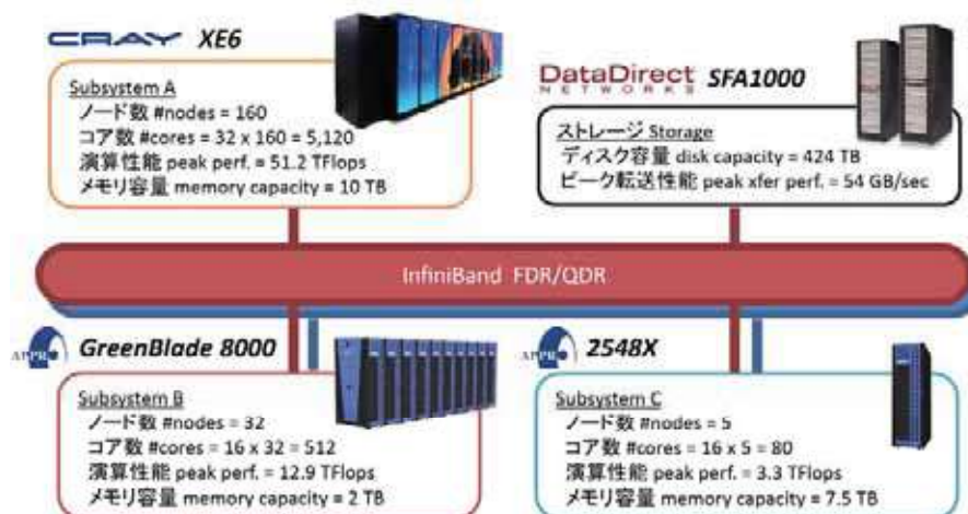
図 1: 電波科学計算実験装置（京都大学学術情報メディアセンターに設置）
