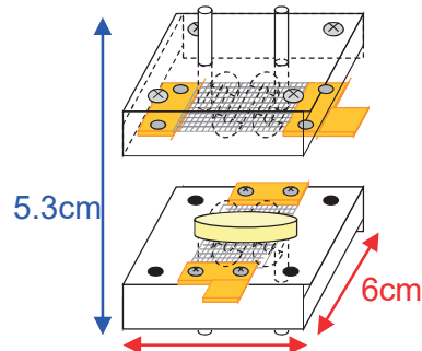
図 1. 新規測定治具
