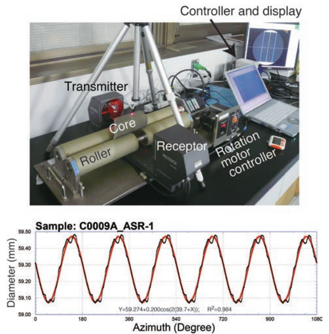
図4 当研究室所有のDCDA法測定装置(上)と測定結果の一例(下)(林ほか, 2017bより改訂)
