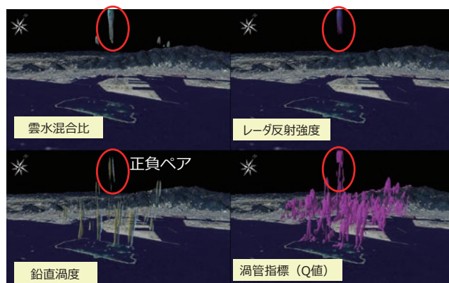
図5 都市気象LESモデルによる積雲シミュレーション
