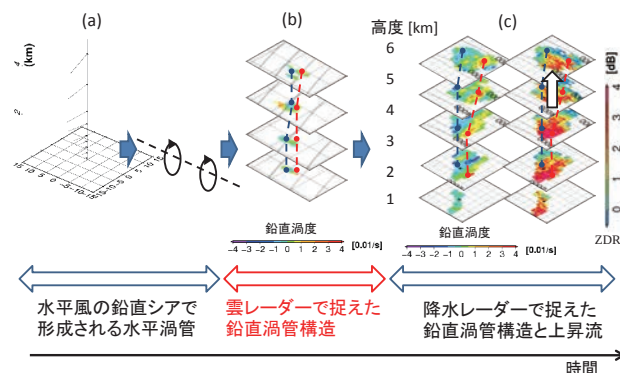
図4 積乱雲内部で渦管構造が形成される様子
