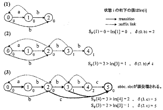
図 8: \text{Oracle}(\text{abbbc}) の誤受理判定
