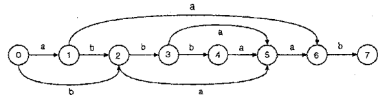
図 1: Oracle(abbbaab)
