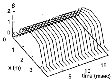
(f) Hall parameter
