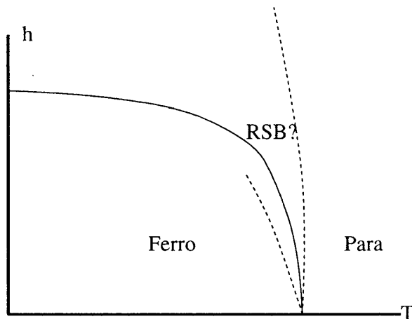
図 2: ランダム磁場 Ising モデルの相図
