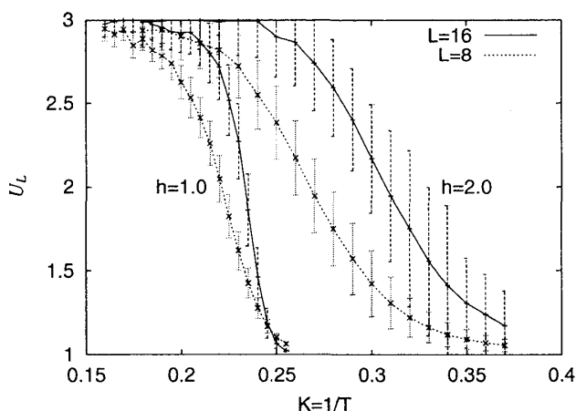
図 3: ランダム磁場 Ising モデルの Binder パラメータ
