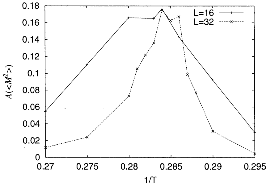
図 1: 希釈 Ising モデル ( p = 0.8 ) の A(<M^2>)
