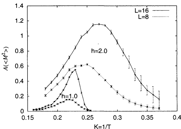
図 4: ランダム磁場 Ising モデルの A(\langle M^2 \rangle)
