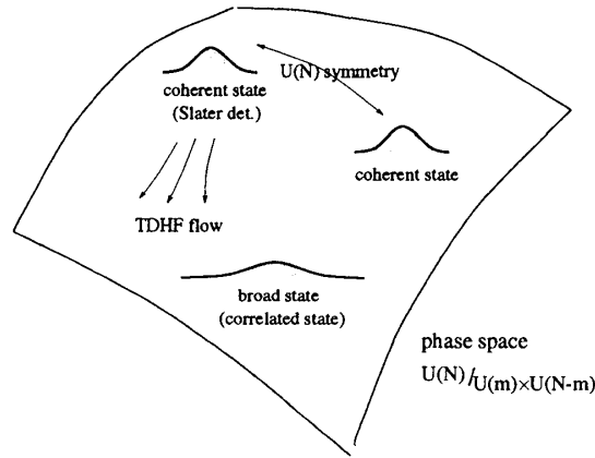
図 1: フェルミオン系の伏見関数の概念図。$N$ 個の一粒子準位に $m$ 個の粒子を詰めた場合、相空間は $U(N)/(U(m) \times U(N-m))$ となる。その上に伏見関数が定義され、最も局在化した波束がスレーター行列式に対応する。この相空間上には、TDHF 方程式による流れが定まっており、この流れのカオス性と、伏見関数の広がりとは、密接に関連しているだろうと予想できる。
