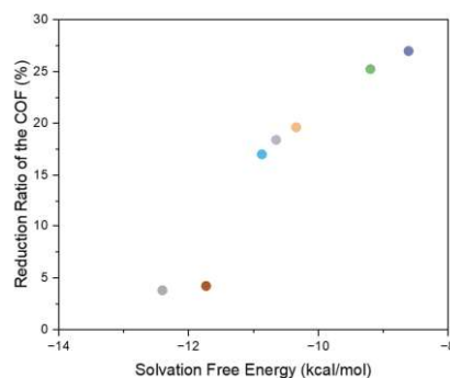
Fig.2 溶媒和自由エネルギーと 摩擦低減率の相関
