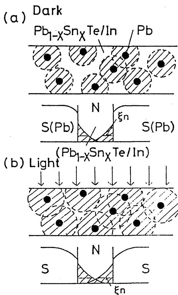
図14 Pb_{1-x}Sn_xTe ; In薄膜中のPb粒による近接効果の模式図。超伝導状態が染みだす様子が斜線部分で表されている。 (a) 光を当てない状態。 (b) 光を照射した状態。染みだしが広がっている。
