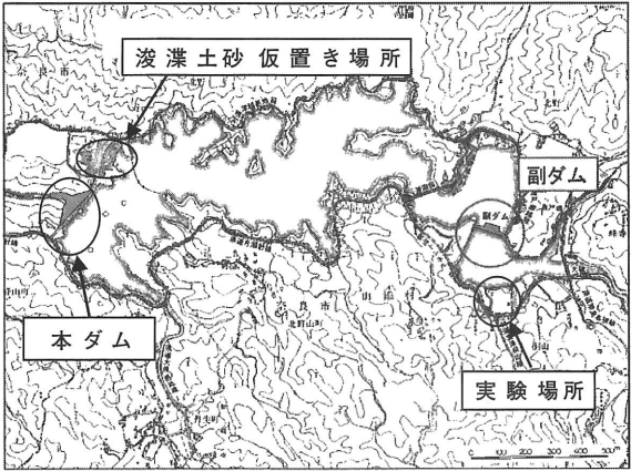
図一4 布目ダムの概要と実験場所
