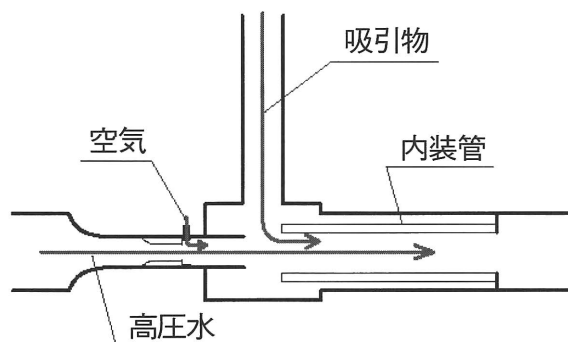
図-1 エジェクターポンプの概念図
