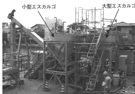
写真-1 スパイラル分級装置（エスカルゴ）
