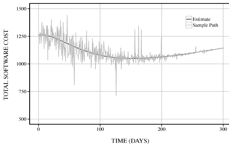
図 3： 推定された総ソフトウェアコスト。
