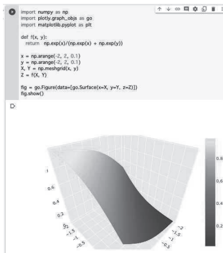
図 4: Softmax function
