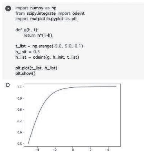
図 3: SciPy:odeint()
