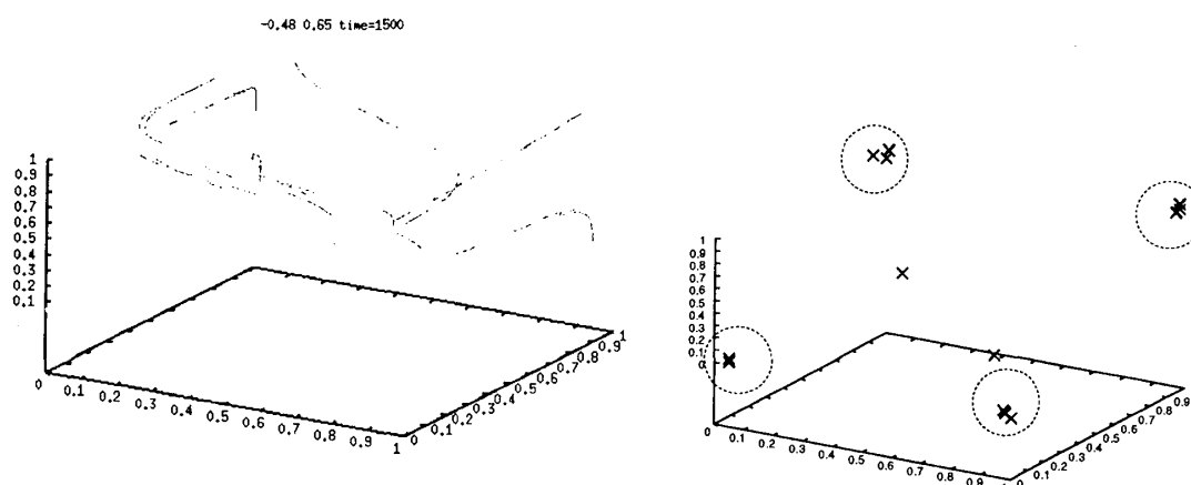
Figure 1: どんな学習をしたかの表示。これは2軸をコンテキストノードの値、1軸をアウトプットノードにとり、ランダムな入力に対する値を順番にプロットしたもので、これをコンテキストプロットと呼ぶ。右側で○で囲んだ部分はオートマトンのノードに対応させられるクラスターを表示。
