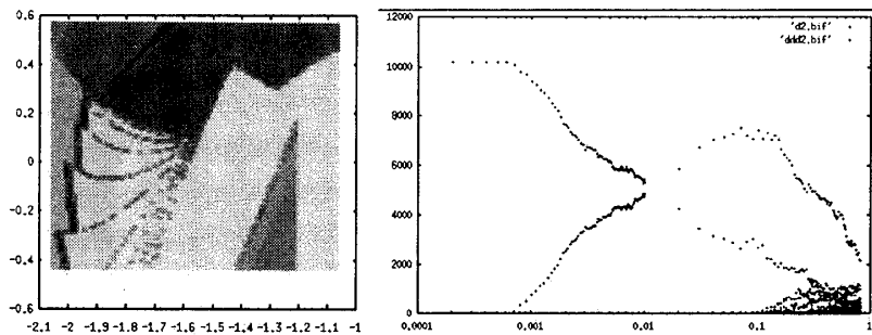
Figure 3: 右側はアトラクターのまわりのベイスン構造。左側はあるアトラクターに収斂したときに最大強度 \sigma でノイズをウェイトにかけて再学習させる。このときに同じアトラクターに戻ってくるか、別なものに収斂するかを判定した。判定には、サンプルに使ったものとは別のサンプル ( L=100 ) を用意し、それに対するアウトプットの違いで判定した。それぞれのアトラクターへ10000回の試行でどのくらいが収斂したかを計算して表している。
