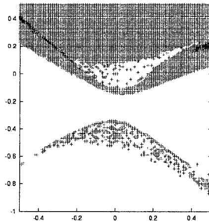
Figure 2: 10000 ステップで学習を打ち切ったときに、答えがeven/odd という形で出せる学習ができた時に学習終了とみなす。初期のウェイト値の空間のある2次元切断面に対し、学習できたか／できないか、がどのように分布しているかを示したのがこの図。点の打ってあるところが学習できた領域で、このうち特に濃い色で点がうってあるところが、空間認識オートマトンに収斂したところである。
