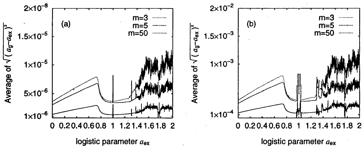
図 平均予測誤差 (推測値 a_g と a_{\text{ex}} の差の平均値). 異なる初期値 x_1 とノイズ列から生成した 100 組のデータ列 \{x_n\} (n = 1, 2, \dots, N) 各々に対して Q(N, a) を最小にする a_g を求めた. a_{\text{ex}} のきざみ幅は 4 \times 10^{-4} . (a) \sigma_{\text{NS}} = 1 \times 10^{-5} . (b) \sigma_{\text{NS}} = 1 \times 10^{-3} .
