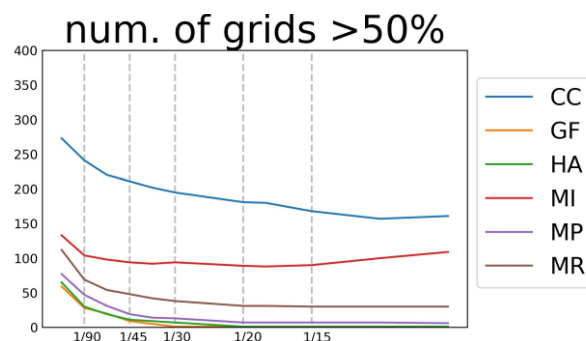
図-6 繰り返し実験における逆転発生割合が 50%を超えるグリッド数。年最大日単位降水量の再現期間（横軸）に対する逆転発生割合が 50%を超えるグリッド数（縦軸）を 6つの SST パターン別に図示。
