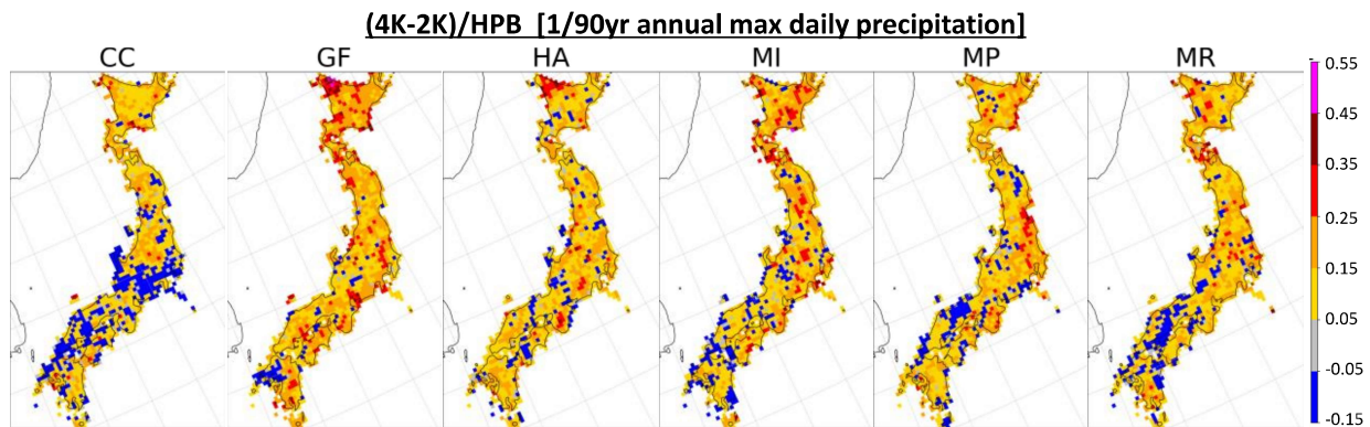
図-2 将来変化倍率差の現在再現実験比. 年最大日単位降水量 (1/90 年) の将来変化倍率の差 (4℃上昇-2℃上昇) を現在再現実験で除した比を 6 つの SST パターン別で推計した結果.
