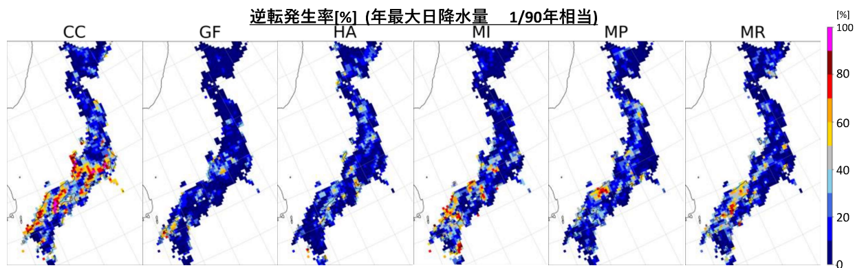
図-5 将来変化倍率に関する逆転発生率。年最大日単位降水量のうち再現期間 90 年に相当するものに関して 2℃上昇実験結果が 4℃上昇実験結果よりも大きくなる割合を繰り返し実験から推計した結果。
