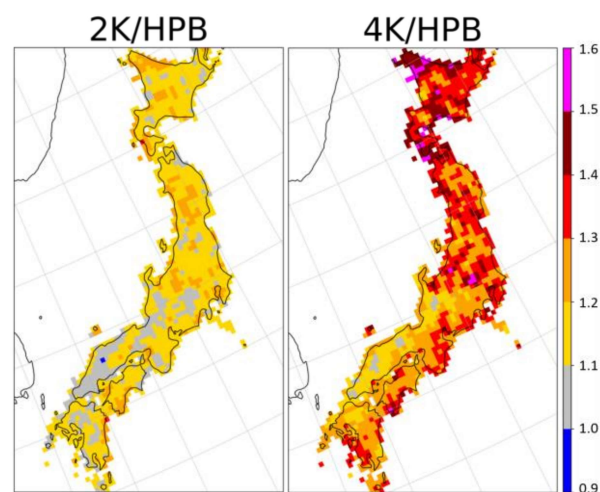
図-1 年最大日単位降水量の将来変化倍率。2℃上昇実験(左図)、4℃上昇実験(右図)における倍率。
