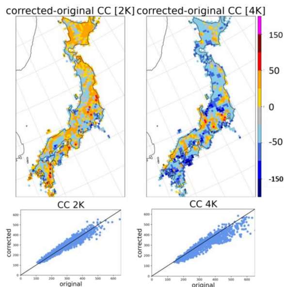
図-7 補正による年最大日降水量の変化 [mm/day]. 年最大日降水量（再現期間 90 年）の補正前後の値を 2℃上昇（左列）、4℃上昇（右列）に関して空間分布（上行）と横軸を補正前、縦軸を補正後とした各グリッドの結果に関する散布図（下行）に図示した。
