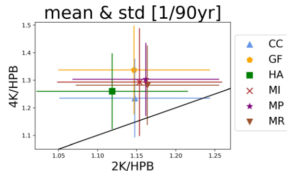
図-4 各 SST パターンの各昇温量における将来変化倍率. 全対象グリッドの平均値が点、標準偏差の幅を線として、2℃上昇時の将来変化量 (横軸) と 4℃上昇時の将来変化量 (縦軸) 上に図示. 両者の倍率が等しくなる点を黒色直線として示した.
