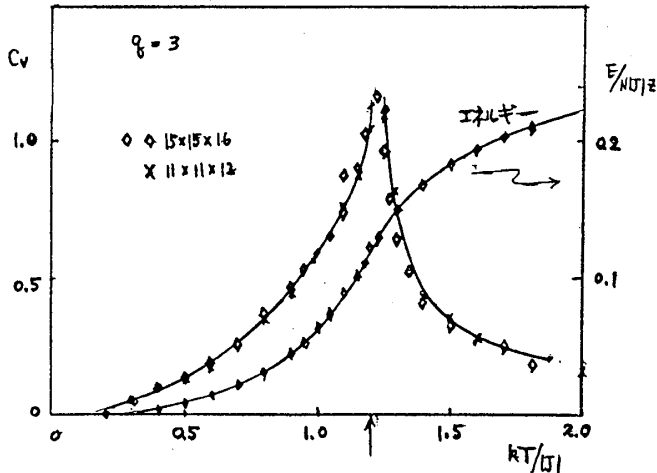
図2. 単純立方格子 q = 3 の比熱の温度変化
