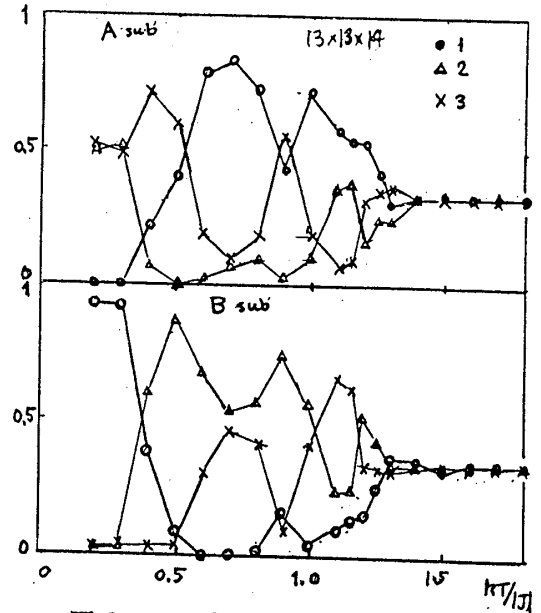
図3. スピン分布の温度変化
