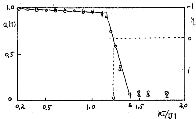
図5. 指数 a(T) の温度変化
