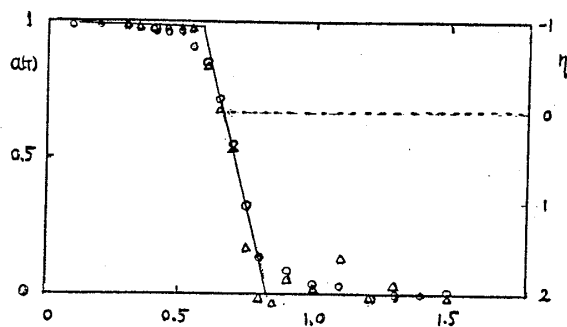
図 9. 指数 a(T) の温度変化
