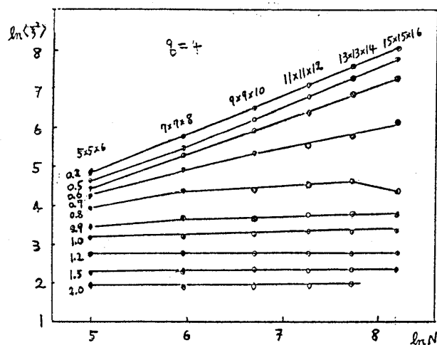
図 8. 秩序変数のゆらぎ
