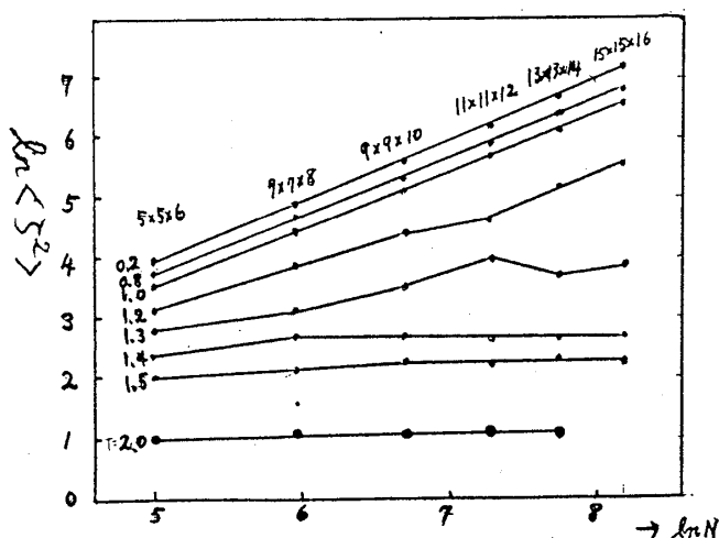
図4. 秩序変数のゆらぎのサイズ依存性
