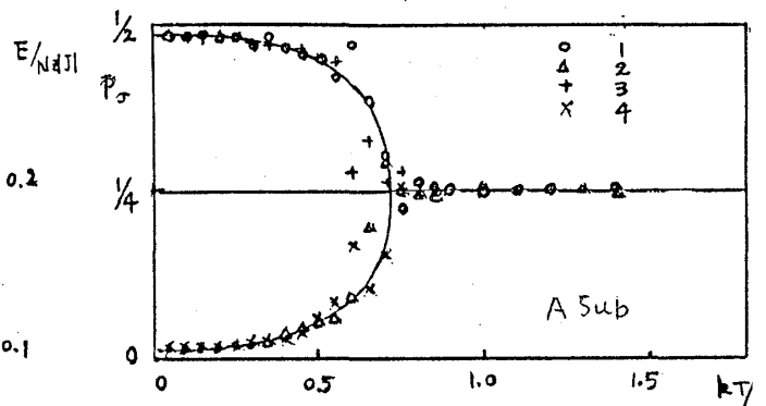
図7. スピン分布の温度変化
