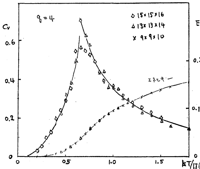
図6. 単純立方格子 q = 4 の比熱の温度変化
