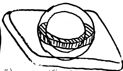
図6. 次元の定義のための概念図
