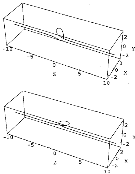
図 4: \Omega = 0.1 (上図が (7), 下図が (11))
