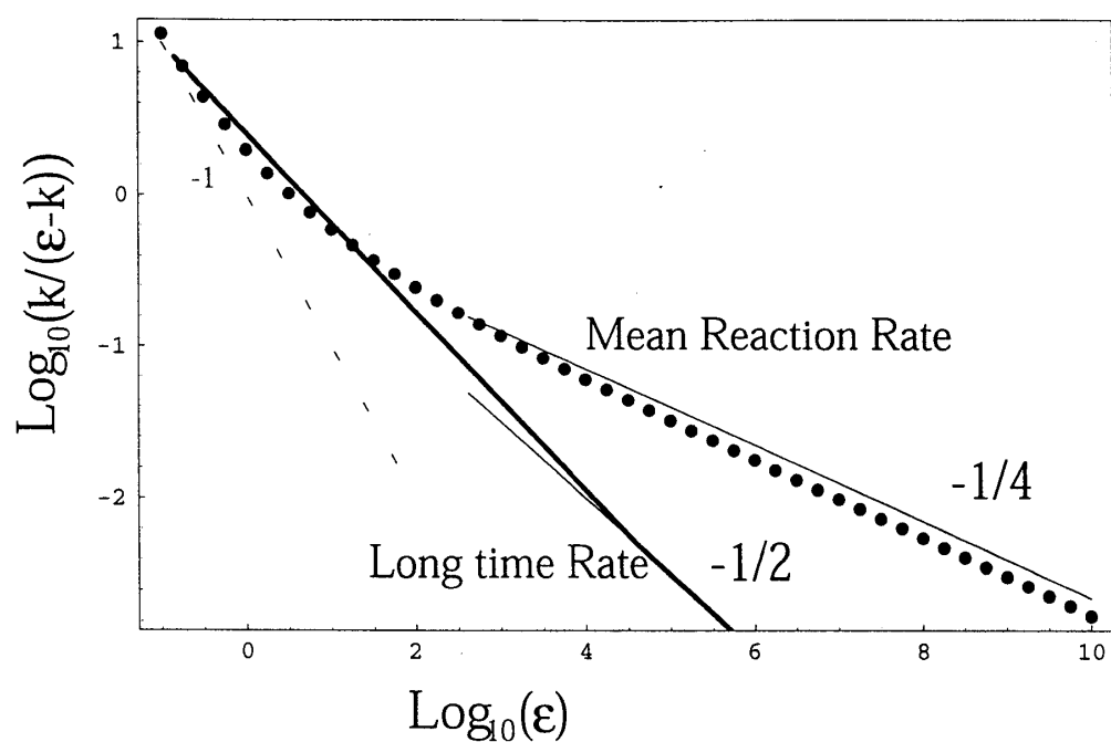
Fig. 1: Zwanzig モデルで反応速度 K/(\varepsilon - K) を \varepsilon に対してプロットした。これは、反応速度を溶媒粘度に対してプロットしたこととほぼ同等である。反応速度としては平均反応速度と長時間反応速度を取り両者を比較している。
