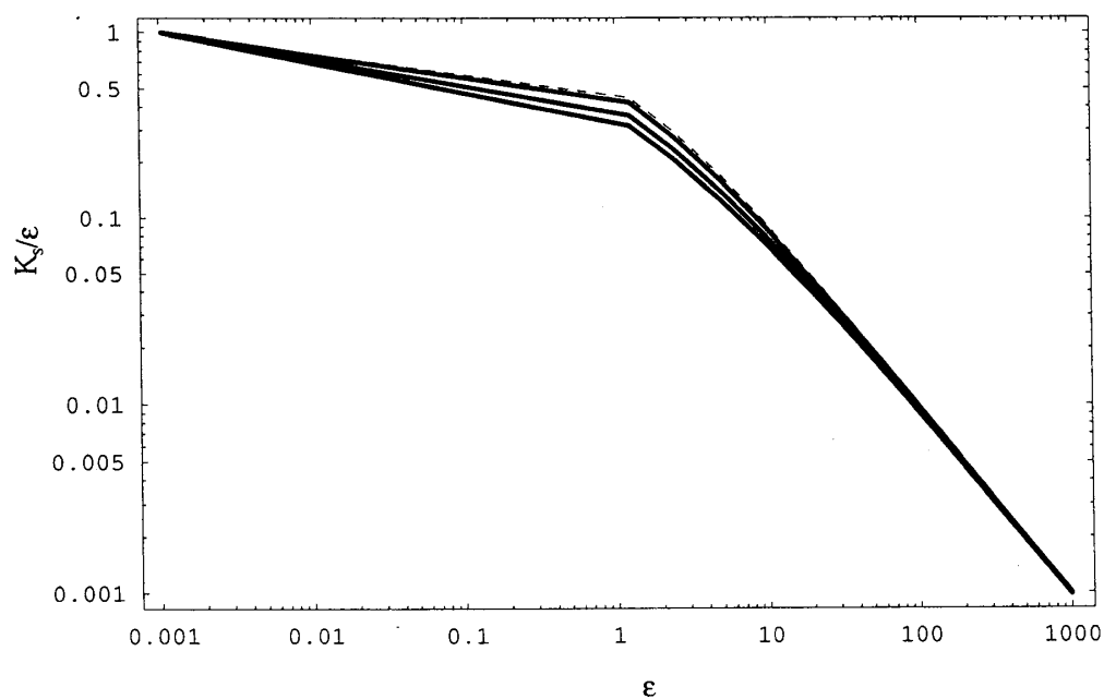
Fig. 2: K_s/\varepsilon を \varepsilon に対してプロットした。反応速度を溶媒の粘度に対してプロットしたことと同等である。 k_D の値は固定されている、 k_D = 1 。ダッシュの線は最低次の近似で \alpha = 0 。線は、上から順に D_r/R^2 = 0.01 , D_r/R^2 = 1 そして D_r/R^2 = 100 。
