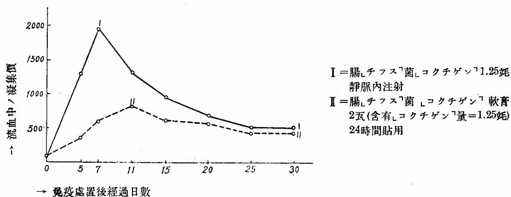
第1圖 各種免疫處置ニヨル血中凝集素ノ推移(第7表參照)
