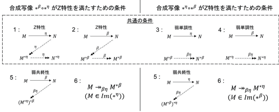
図 5: 定理 15 による 2 通りの Z 定理証明
