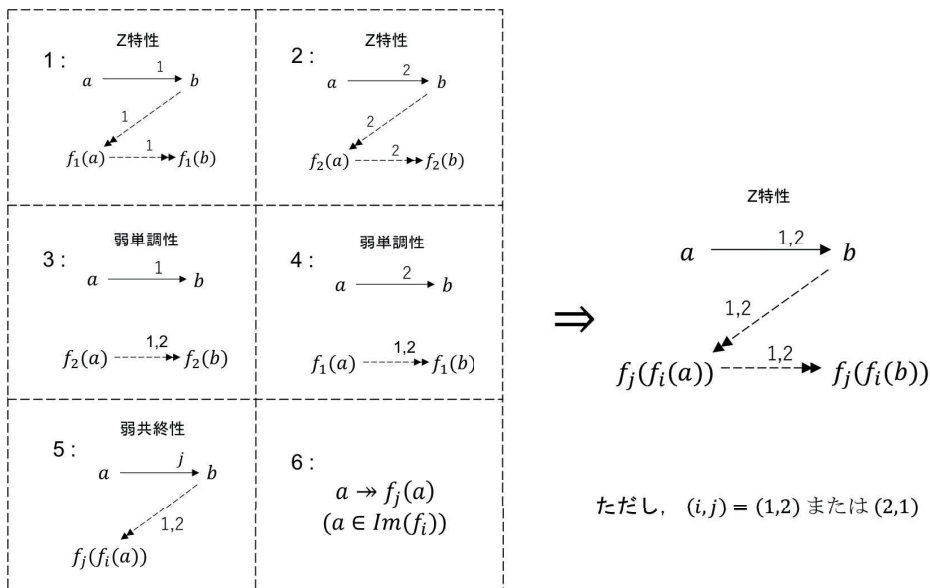
図 4: 定理 15(Z 特性のモジュール性)
