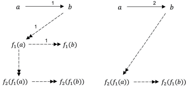
図 3: 合成的 Z 定理
