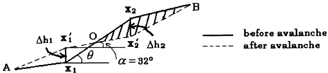
Fig.4 Sand avalanche
