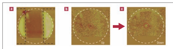
図3 磁気コア反転のMFM観察結果 a: 試料の原子間力顕微鏡像。円形の白破線内が磁性ナノドット。 b, c: 電流印加前後の磁気力顕微鏡像。
