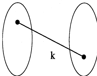
図 2. 原子
