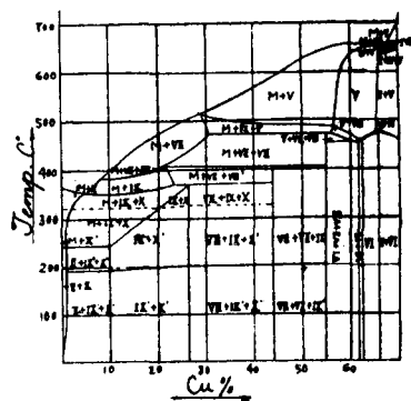
Fig. 12 Parallelschnitt 30% Sb
