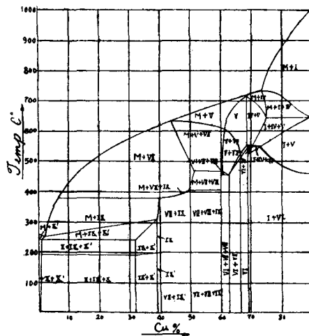
Fig. 8 Parallelschnitt 10% Sb
