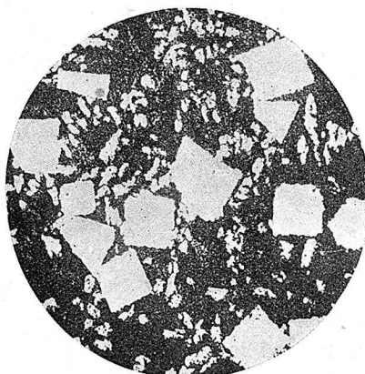
Photo 17. 5%Cu, 10%Sb, 1%Pb und 84%Sn
