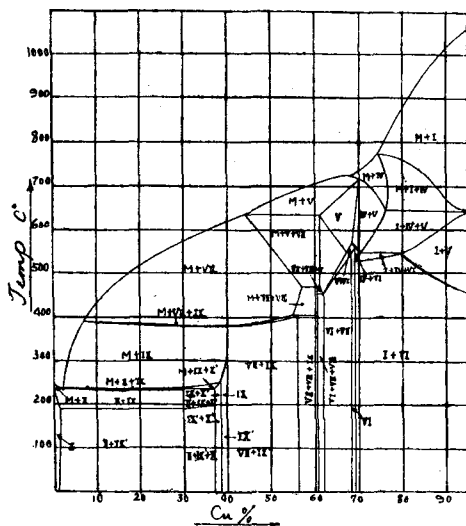
Fig. 7 Parallelschnitt 5% Sb
