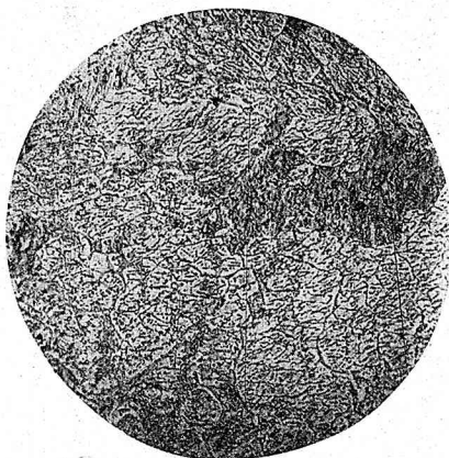
Reg. mit 65%Cu, 10%Sb und 25%Sn, bei 400° geglüht: VI+VII. 100 Verg.
