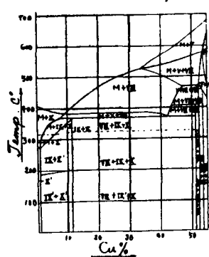
Fig. 15 Parallelschnitt 45% Sb
