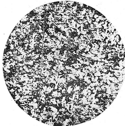
7%Cu, 7%Sb und 86%Sn
