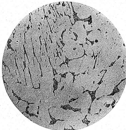
Reg. mit 60%Cu, 30%Sb und 10%Sn, bei 400° geglüht: VI+VIII+VII. 100 Verg.
