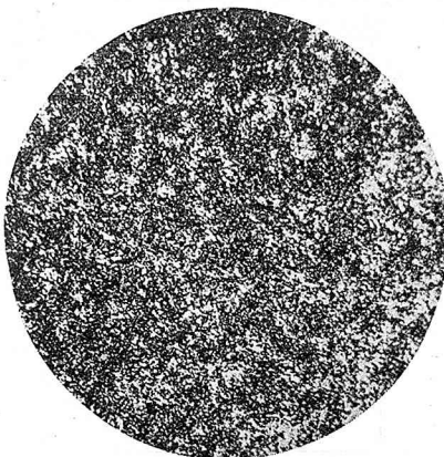
Photo 18. 3%Cu, 4%Sb und 93%Sn
