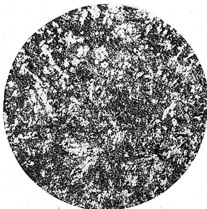
Photo 15. 5%Cu, 4%Sb und 91%Sn
