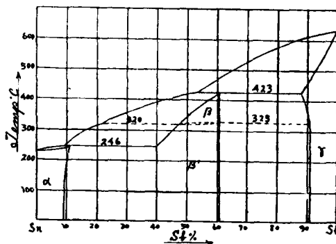
Fig. 2 Zinn-Antimon
