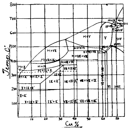
Fig. 10 Parallelschnitt 20% Sb
