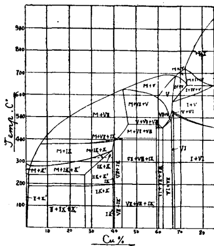
Fig. 9 Parallelschnitt 15% Sb
