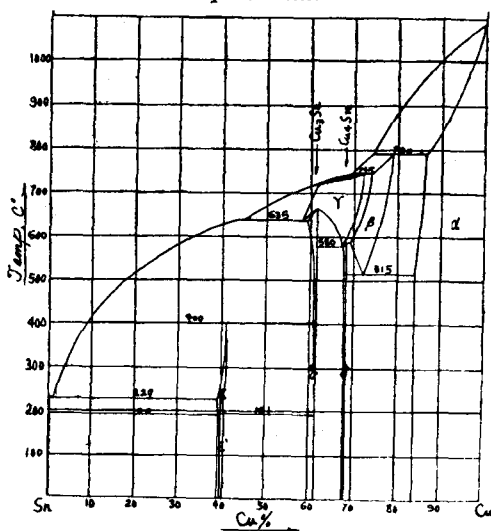
Fig. 1 Kupfer-Zinn
