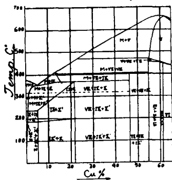
Fig. 16 Parallelschnitt 50% Sb
