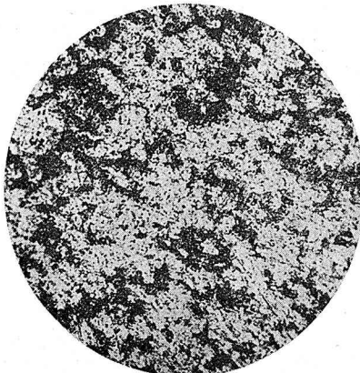
7%Cu, 4%Sb und 89%Sn
