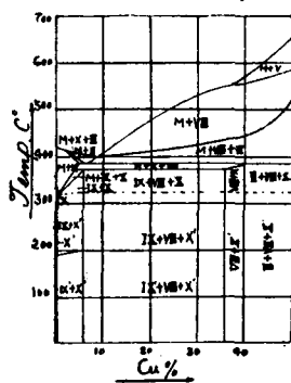
Fig. 16 Parallelschnitt 50% Sb
