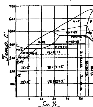
Fig. 14 Parallelschnitt 40% Sb
