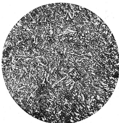
Photo 16. 5%Cu, 7%Sb und 88%Sn
