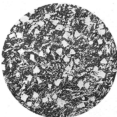
Photo 14. 7%Cu, 10%Sb und 83%Sn
