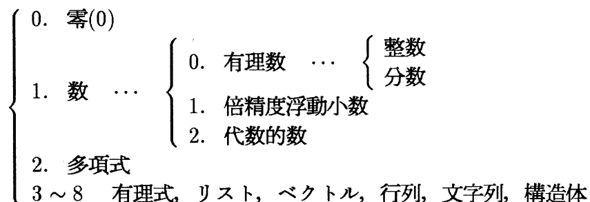
Fig. 1. risa/asir のデータ構造
