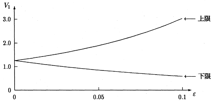
(a) 区間演算 (数値計算)
