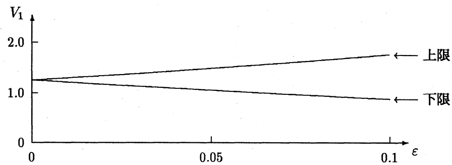
(c) 記号解 (4) に代入した場合
