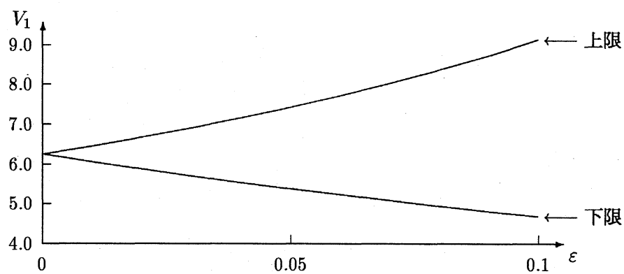
(a) 区間演算 (数値計算)
