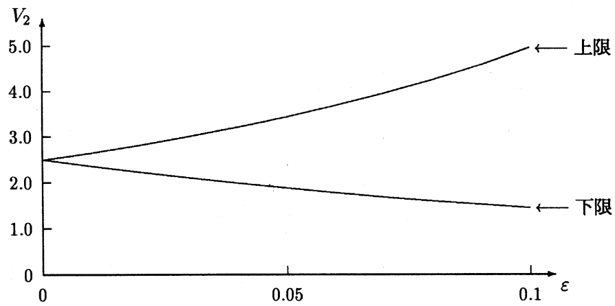
(a) 区間演算 (数値計算)
