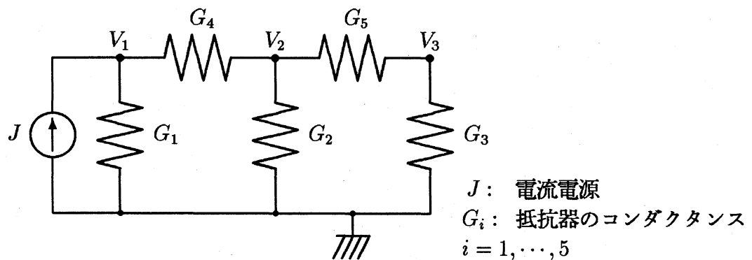
Fig. 3. 梯子型抵抗回路
