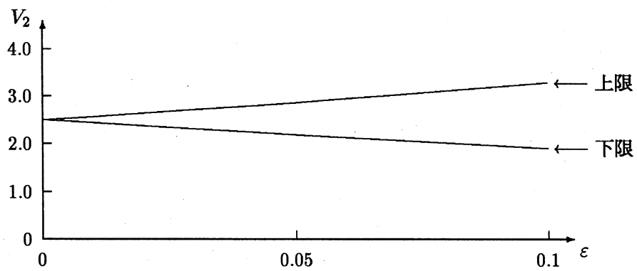
(c) 記号解 (4) に代入した場合
