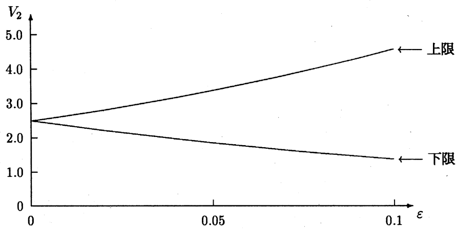
(b) 記号解 (3) に代入した場合
