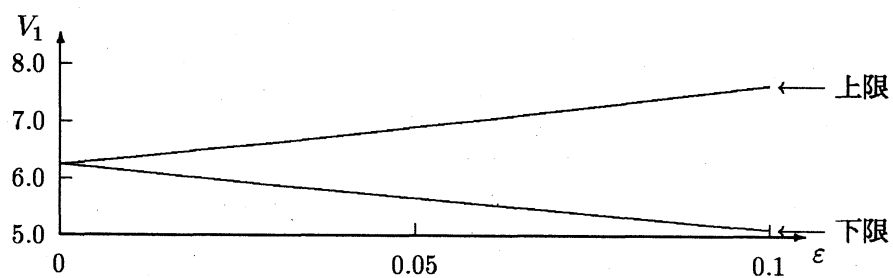
(c) 記号解 (4) に代入した場合
