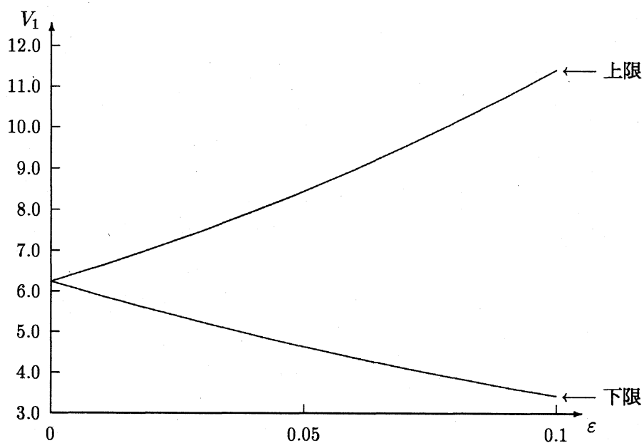
(b) 記号解 (3) に代入した場合
