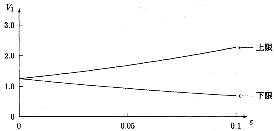
(b) 記号解 (3) に代入した場合
