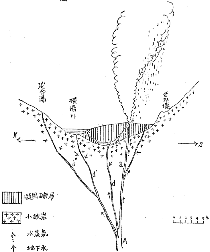
地獄谷噴泉地下想像斷面模式圖
