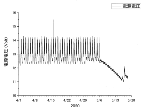
図.5 電源電圧モニタリング
