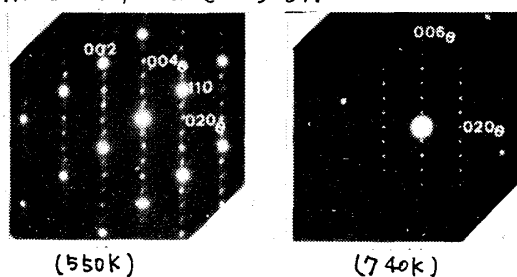
図2. 図1に対応する領域からの電子回折図形
