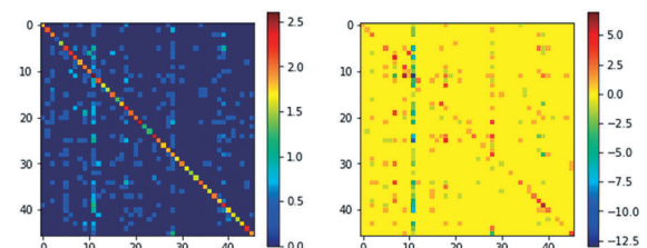
図4. 混同行列
