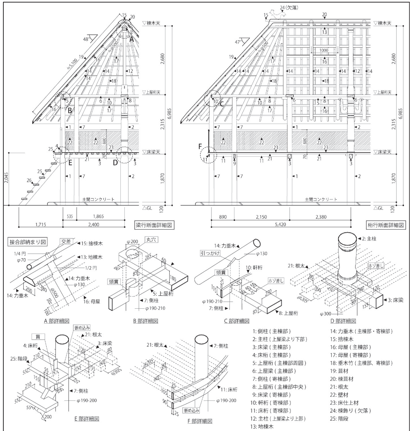
図3 TQ社 断面詳細図・接合部詳細図
