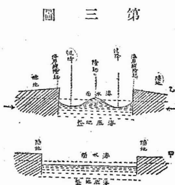
第三圖 相模灣底に於ける隆起 昇降運動假想圖
