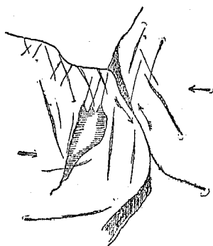
敦賀灣東岸の著しい斷層崖の直下に於ける深い海底の切込は、充分斷層地形を思はしめ南々東に琵琶湖の東岸となり、不破關附近に至り該線は少し東部へ彎曲をなし夫より急に南東に走つて養老山脈の東崖をなしてゐる。此處にも等しい三角崖をなし新しい斷層崖を現してゐる。又其後部に當る鈴鹿山脈の東崖も同様であつて共に、東部に隆起せる傾動地塊である。此外京都盆地の西に於ける龜岡盆地をなせる東部の山崖
