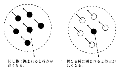
図 2: 左図: 同じ種の個体に囲まれたとき得点が高い. 右図: 違う種の個体に囲まれたとき得点が低くなる.
