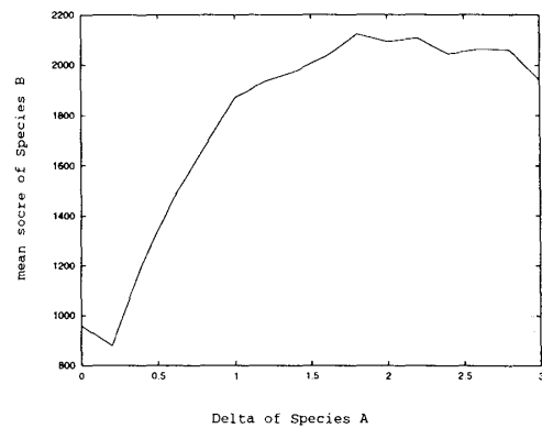
図 9: 横軸は、種 A の \Delta_i の平均で、縦軸は種 B の平均得点 (全ての平均 \Delta_i で平均したもの)。種 A の平均 \Delta_i が 0 に近いとき、種 B の平均得点は低くなる。
