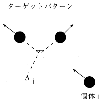
図 1: 左上の 2 個体の頭の相対角度が \Delta_i のとき, 右下の i 個体はその方向に向かう. このとき, 左上のペアをターゲットパターンという.
