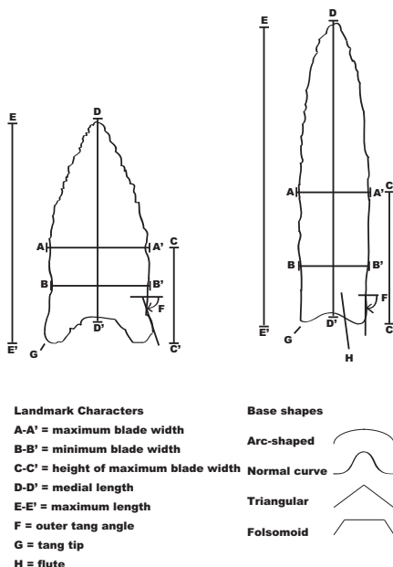
図 2 O'Brien et al. (2001) p. 1127 から、矢じりの各部位に注目して形質をコード化していく。実際にどのような基準でコード化するのかは、次の図を参照。
