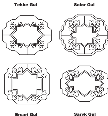
図 4 Tehrani & Collard 2002, p. 449 から．このような模様の有無を 0 と 1 という値に変換し，様々な模様の有無に基づく行列を用いて系統樹が作成される．
