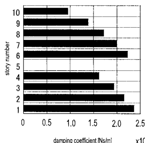
図 2. 最適ダンパー配置
