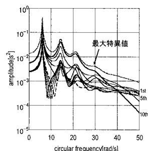
図 3 付加ダンパーを配置しない場合の層間変位伝達関数振幅と最大特異値
