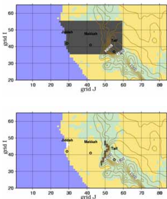
図 1：数値モデル中での緑化領域（灰色）。(a) はジェッダ、メッカ、タイフを含む 100km × 150km、(b)は山岳地域の 100km × 10km。
