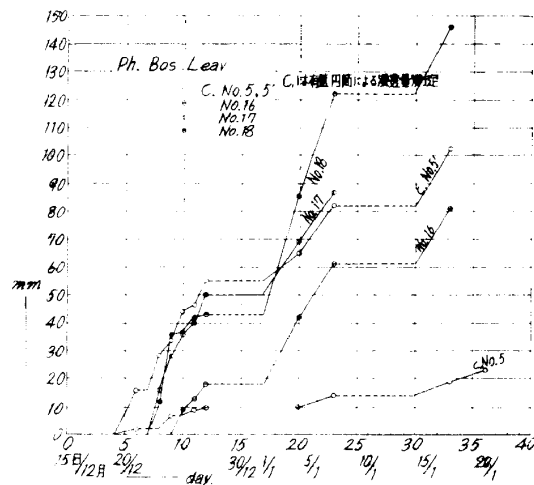
図-3 乾季稲水田の減水深観測値
